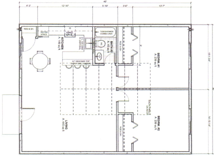
1 FLOOR PLAN SCALE: 1/8" = 1'-0"
